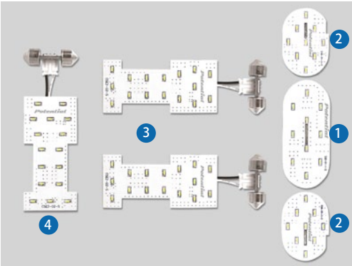
①フロントルームランプ ②フロントマップランプ ③サイド・リアルームランプ ④ラゲッジランプ
