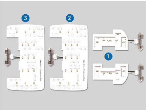
①フロントルームランプ ②センタールームランプ ③リアルームランプ
